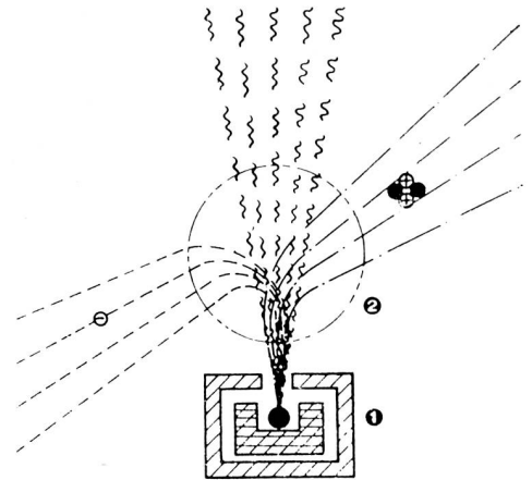
Fig. 4 Strahlendes Radiumpräparat (1) im Magnetfeld (2). Durch das Magnetfeld lassen sich die 3 Strahlenarten \alpha -, \beta - und \gamma -Strahlen abbiegen und trennen.
