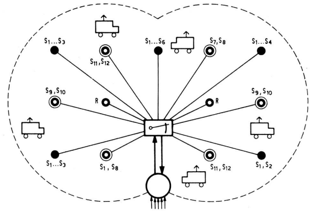
Fig. 1 Prinzipieller Aufbau eines Autotelephonnetzes mit 1 Rufkanal R und 12 Sprechkanälen S_1 \dots S_{12} (zugeteilte Kanalnummern frei gewählt)
