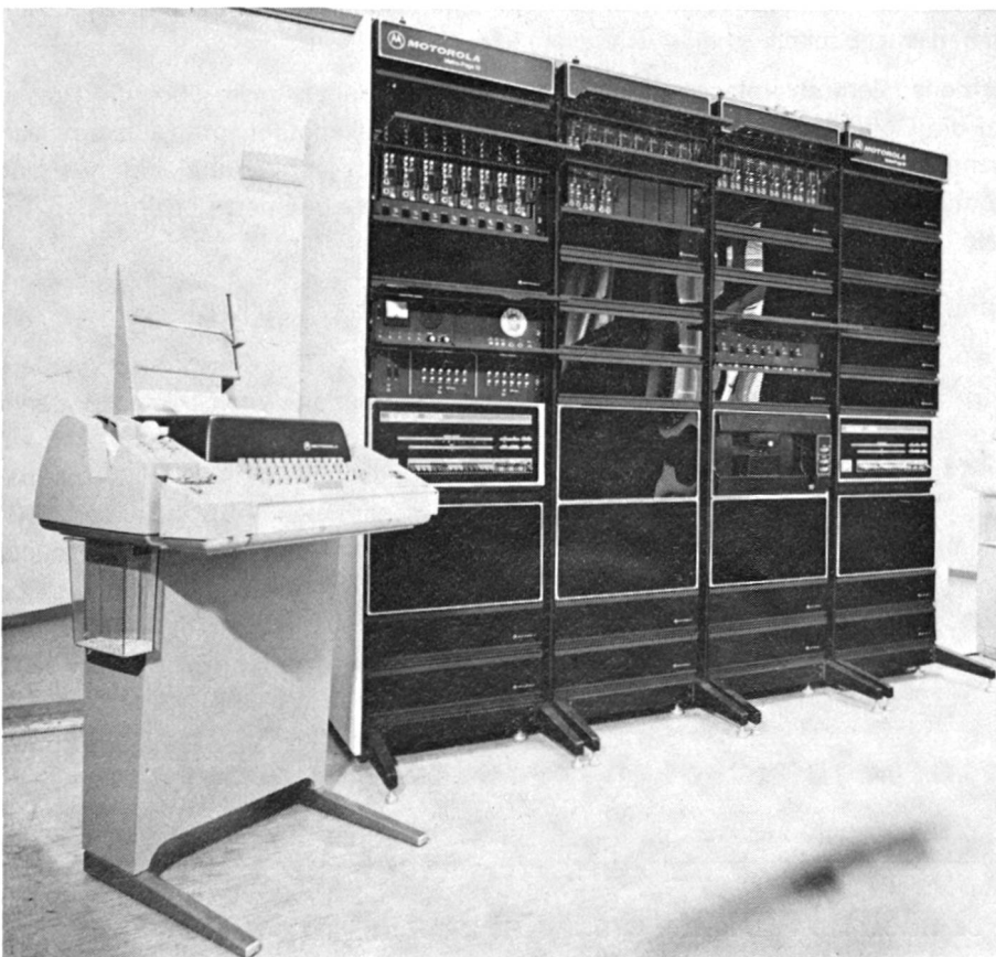
Die Ueberleiteinrichtung ist das Herz der Anlage. Links im Bild ist der Systemfern-schreiber sichtbar, in der Buchst. 1 und 4 befinden sich die beiden Zentralrechner
