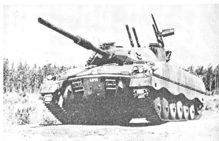
Le IKV (Infanteriekanonvagn) 91 est destiné à remplacer, dans les brigades d'infanterie et les brigades NORRLAND, les canons automoteurs de 105 mm anciens.
