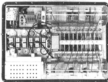
Der Blick ins Innere des Antennentuners ATM1000 zeigt die binär gestuften Spulen und Kondensatoren.
