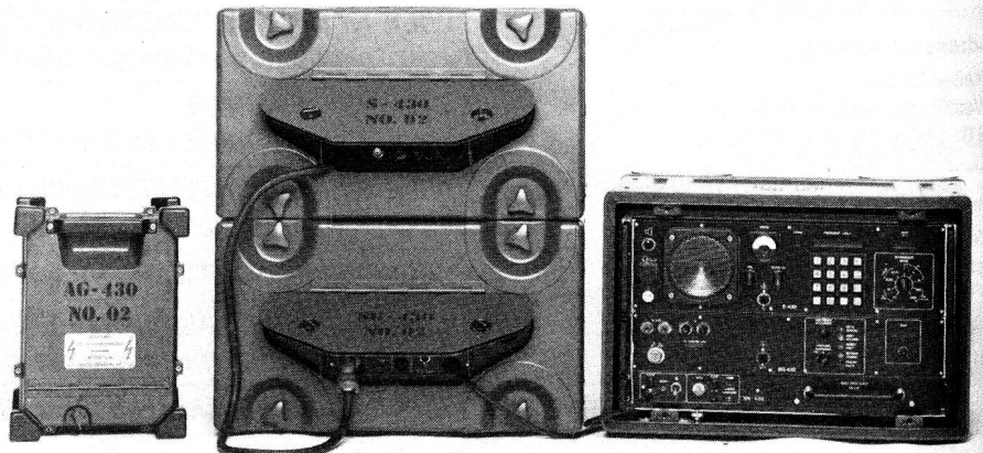
Die Funkstation SE-430 besteht aus (v.l.n.r.): Antennenabstimmgerät, Sender und Speisegerät, Empfänger (inklusive Bedienungseinheit).
