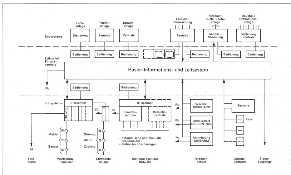
Abb. 1 Schematischer Aufbau des Alarmmanagement-Systems
