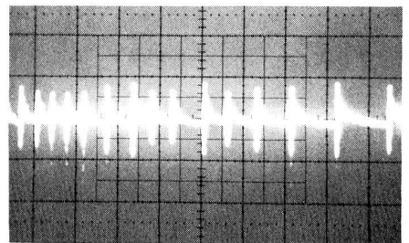
Bild 3 Einschaltstörungen an der gleichen Armatur wie Bild 2. Zeitlicher Verlauf der Gegenaktstörspannung auf dem 220-Volt-Netz. Gemessen zwischen Phase und Nulleiter (Massstäbe: 50 Volt und 10 Mikrosekunden pro Einheit).
