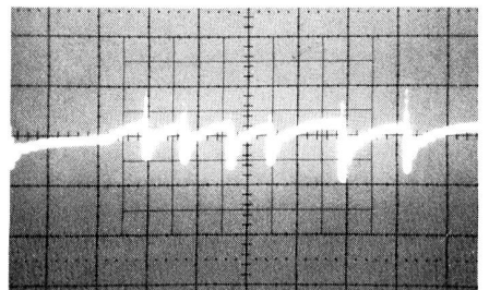
Bild 4 Einschaltstörungen an der gleichen Leuchtstoffröhrenarmatur wie Bilder 1 und 2. Gleichaktstörspannung auf dem 220-Volt-Netz, gemessen zwischen Phasen- und Schutzerdungsleiter (Massstäbe: 50 Volt und 10 Mikrosekunden pro Einheit).
