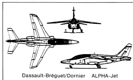
Dassault-Breguet/Dornier ALPHA-Jet
