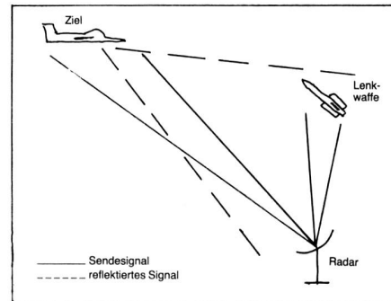
Funktionsskizze für BL-64.
