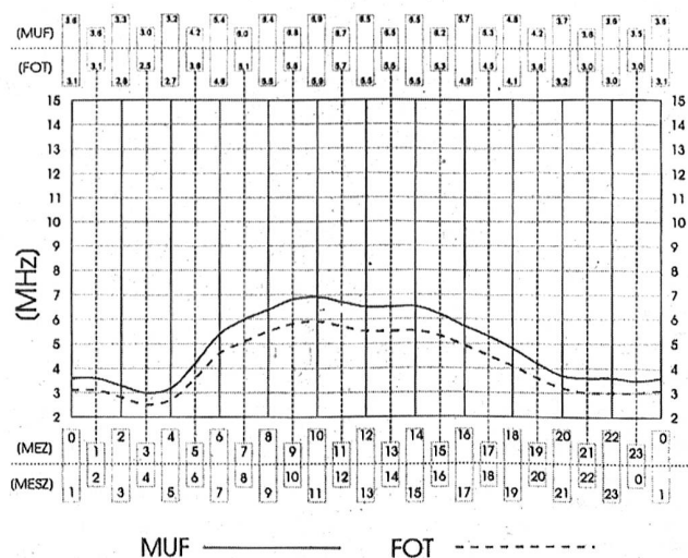
Bern OKTOBER 1996 R = 5
