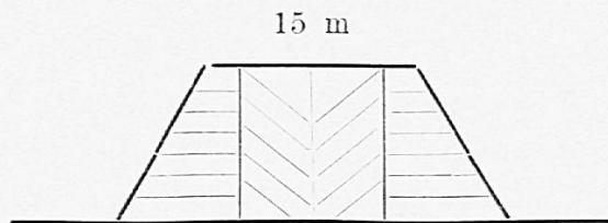
Fig. 23. Querschnitt.
