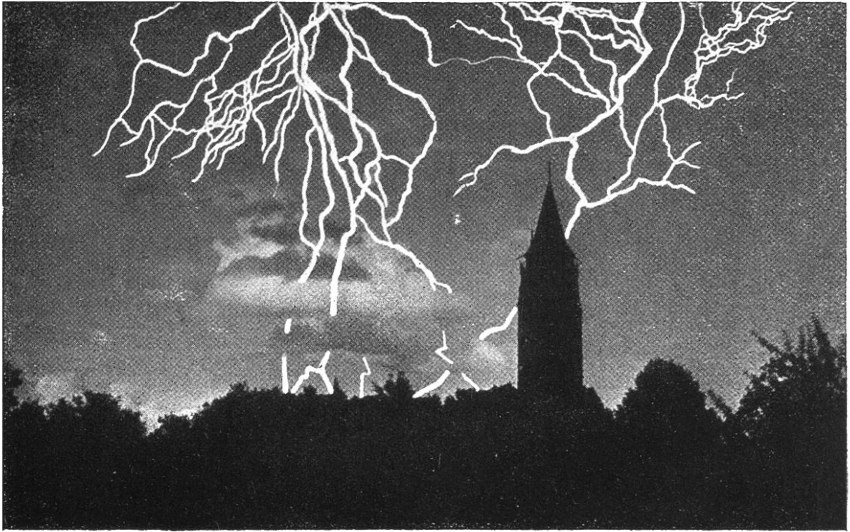
PHOTOGRAPHISCHE AUFNAHME EINES BLITZES BEI NACHT ::
