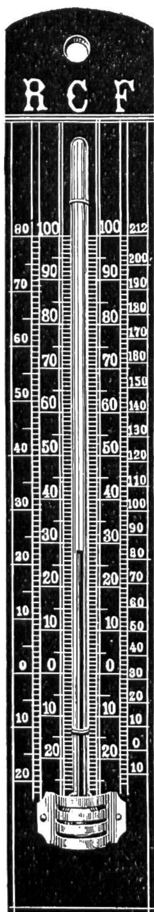
Réaumur-Celsius-Fahrenheit
