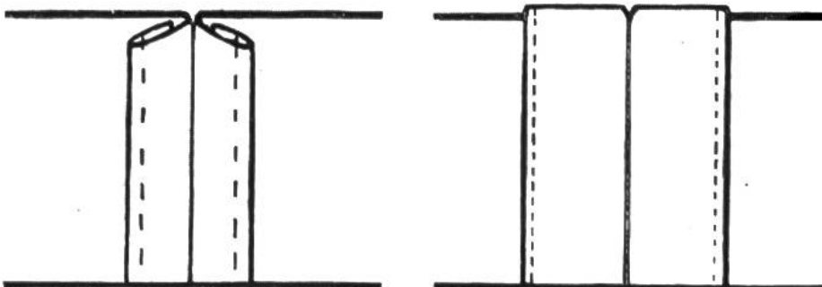
Nähte an Trikot-Stoffen, links 2. Art, rechts 3. Art.
