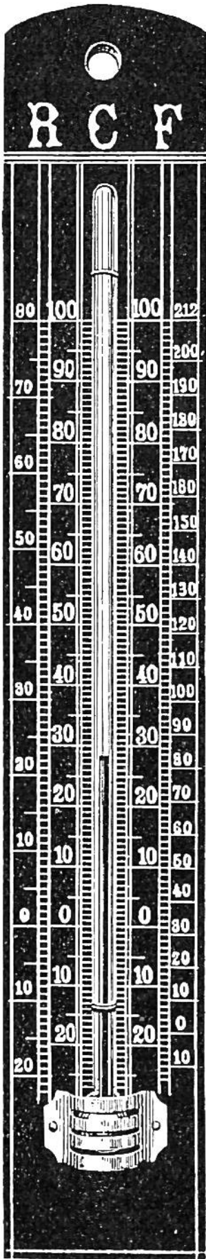
Réaumur-Celsius-Fahrenheit
