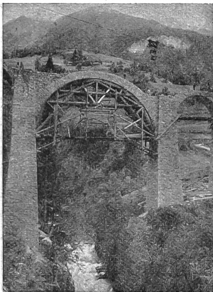
Grosser Bogen des Grenchols-Viadukts (Wallis) im Bau (1912). Die auf dem Viadukt befindlichen Arbeiter bilden einen Masstab für die Grösse des Baues.
