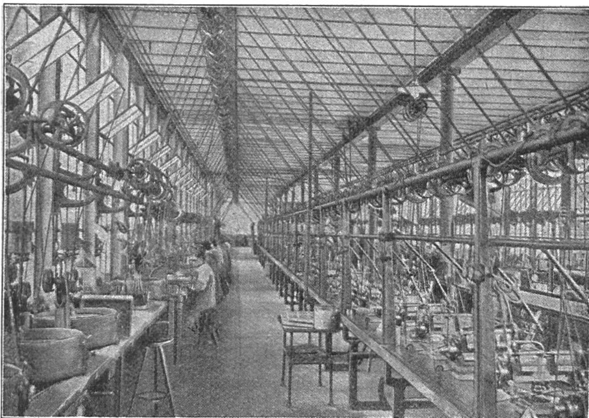
Teilanfsicht eines Arbeitsraumes „Zenith“ für Stahlstücke.
