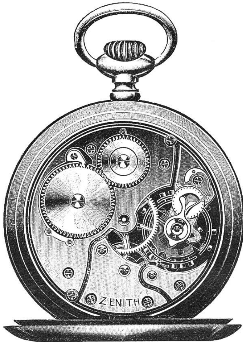
Uhrwerk einer Taschenuhr „Zenith“.
