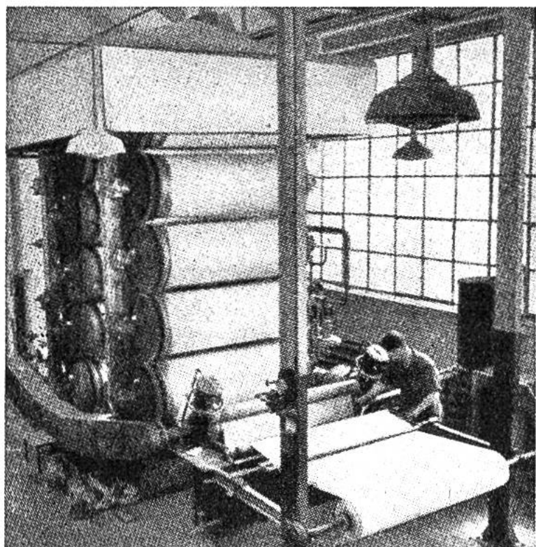
Das Stoffband läuft über die Walzen der Imprägniermaschine; dabei wird auch das feinste Fäserchen von der flüssigen Gummimilch durchtränkt; dies soll verhindern, dass beim Gebrauch zwischen den Fäden Reibung und dadurch dem Pneu schädliche Hitze entsteht.
