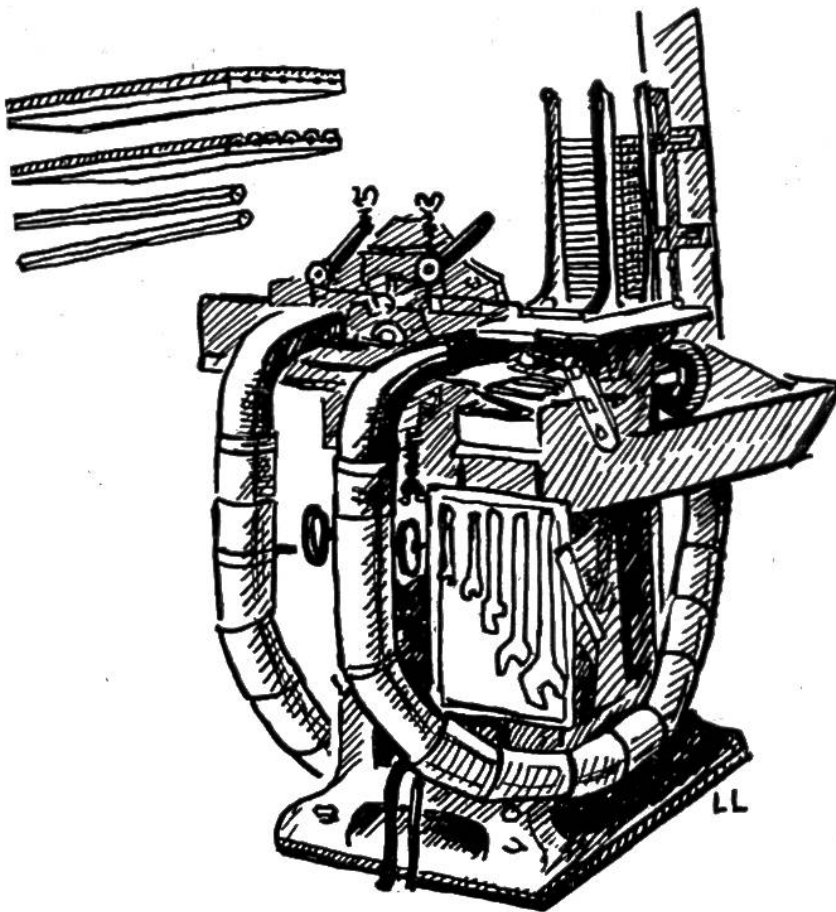
Die automatischen Aushobelmaschinen beenden die Umwandlung der Cedernholz - Brettchen in Bleistifte.
