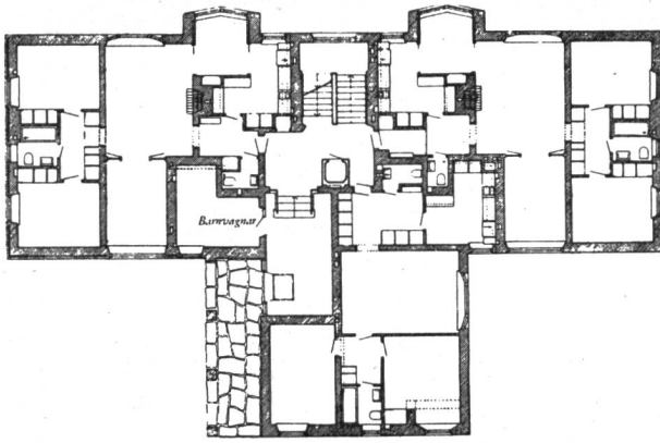
Abb. 6. T-Haus-Grundriss aus der Siedlung Guldheden bei Göteborg. Erdgeschoss: zwei 4½-Zimmerwohnungen, eine Dreizimmerwohnung. Schlafzimmer, Bad- und Arbeitszimmer gefangen. Arch. Wejke und Oedeen.
