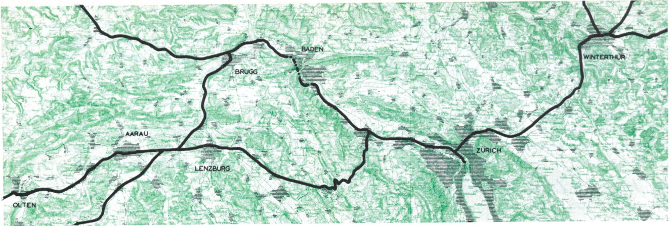
Abb. 7. Die Durchgangsstrassen im Raume Olten—Winterthur nach dem offiziellen Ausbaurvorschlag.
