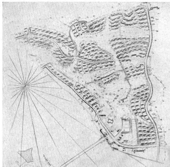
Abb. 28. Siedlung bei Beersheva, in wüstenartigem Klima; Erstellung auf welligem, durch tief eingeschnittenen Wadis unterbrochenem Gelände, mit Raum für 5000 Einwohner; alle Wohnstätten sind nach vorherrschenden Winden orientiert.
