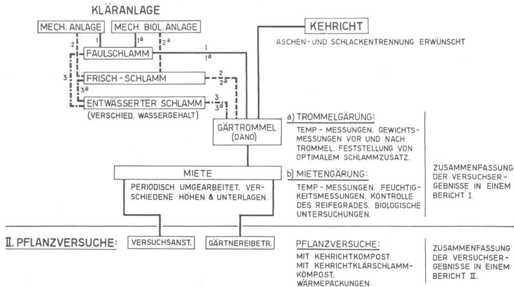
Abb. 1. Kehrriichtaufbereitungsanlage Rüschlikon: Schema der Versuche.
