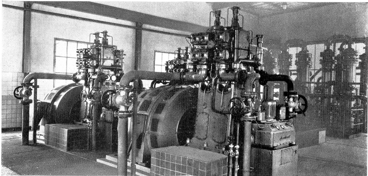
Kompressorstation der Gasfernleitung Saarbrücken-Paris
