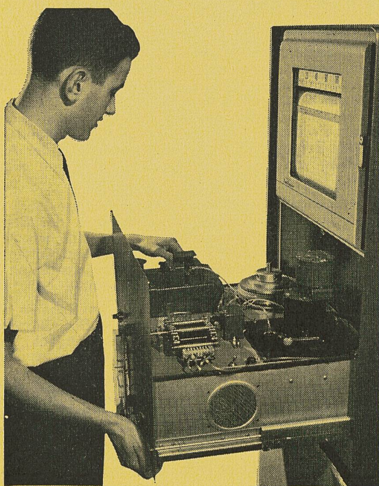
Bewegliches Apparatesystem
