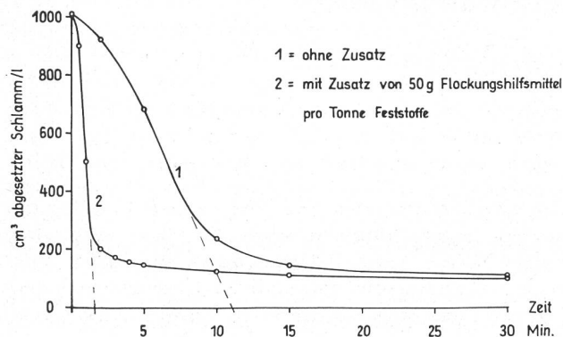
Abb. 1. Absatzkurven für Kieswaschwasser bei pH 8,0 mit und ohne Flockungshilfsmittel.
