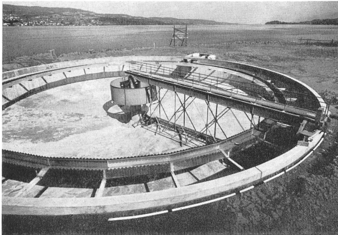
Kläranlage Horgen
