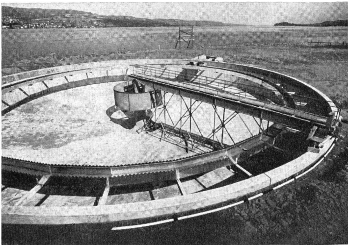
Kläranlage Horgen
