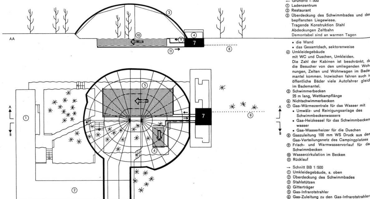
Abb. 5. Grundriss und Schnitt durch das Zelthallenbad in Lommerbergen
