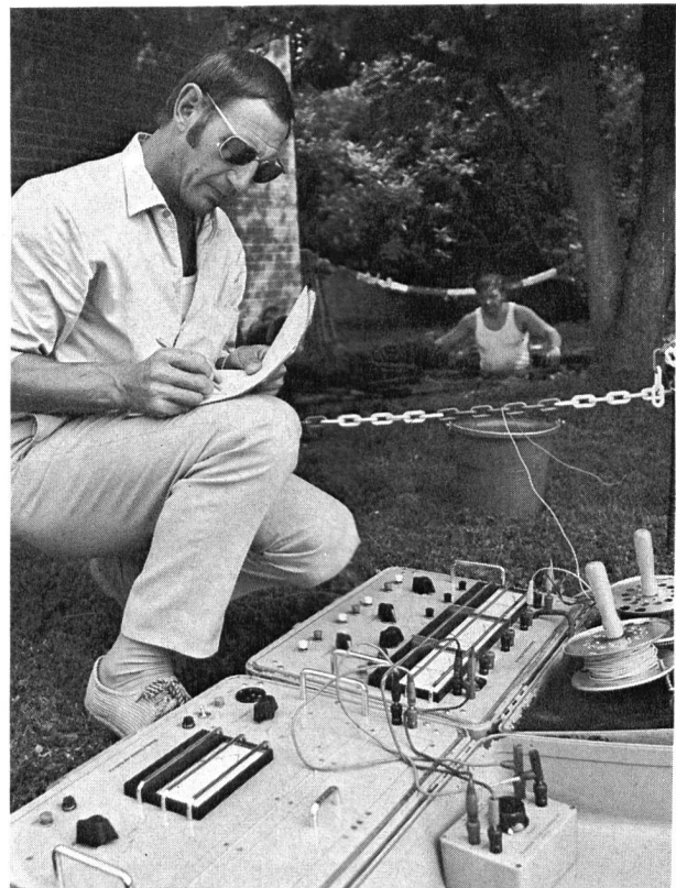
Potentialmessung eines erdverlegten Heizöltanks. Im Arbeitsumfang unserer Tankrevisionen inbegriffen
