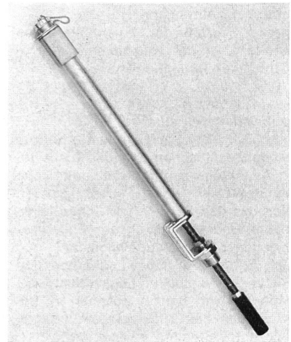
FD 7-SR für erdverlegte Tanks (bis etwa 1 m Domschachtiefe)
