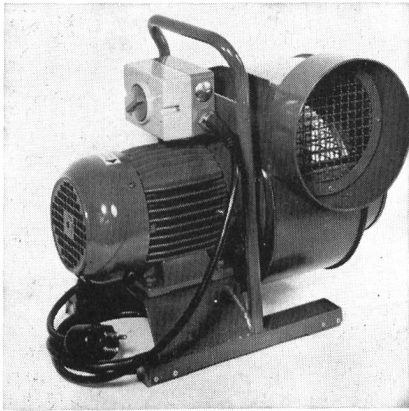
Normale Ausführung 40 und 60 m³ Leistung pro Minute. In 220 oder 380 Volt lieferbar.
