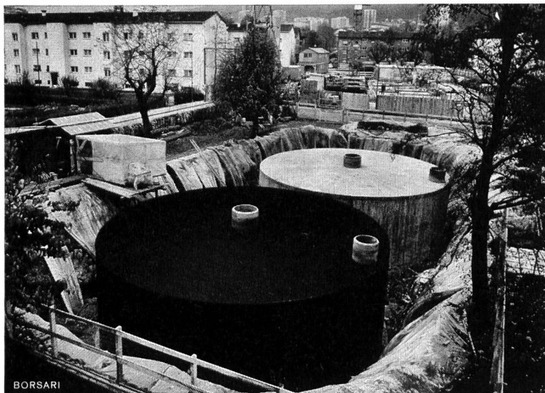
Gemeinnützige Baugenossenschaft Limmattal, Zürich 2 Tanks, total 1 000 000 Liter Heizöl
