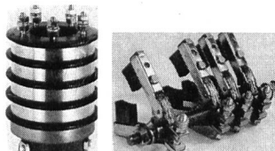
Schleifringkörper und Bürstenhalterelemente auch als Sonderausführungen
