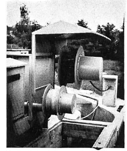
Federkabeltrommel als Längsstromzuführung an einem Längsräumler in einer Kläranlage, Kabelzug horizontal
