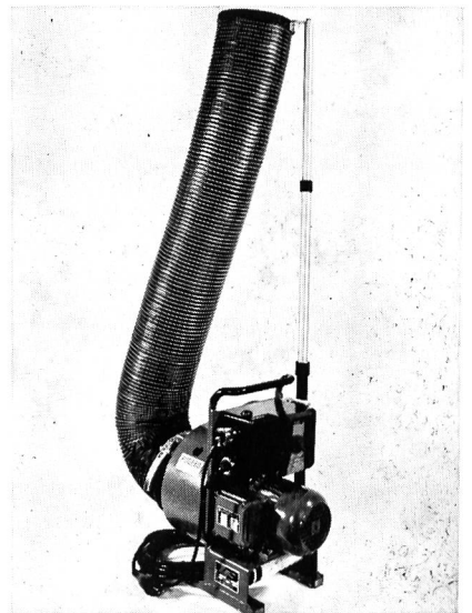
Stativ Ideal zum Belüften von Tanks. Ansaug- höhe der Frischluft: 1,5 m ab Boden. Die Halterung ist ausziehbar und lässt sich nach Gebrauch bis zur Höhe des Gerätes zusammenschieben. ▶
