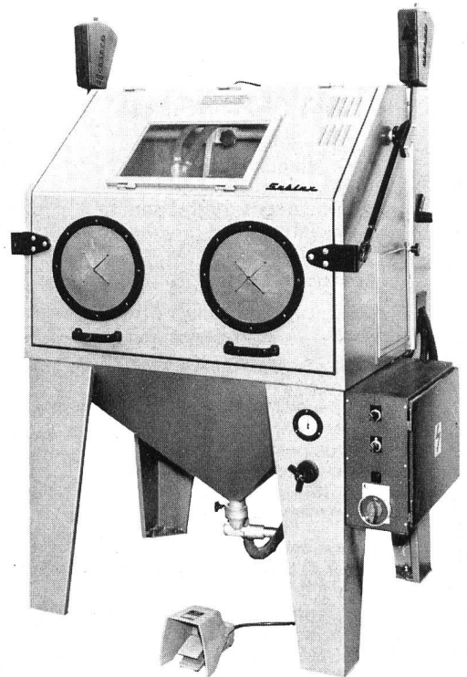
Sandstrahlkabine SABLUX 100
