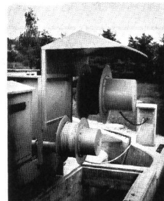
Federkabeltrommel als Längsstromzuführung an einem Längsräume in einer Kläranlage, Kabelabzug horizontal
