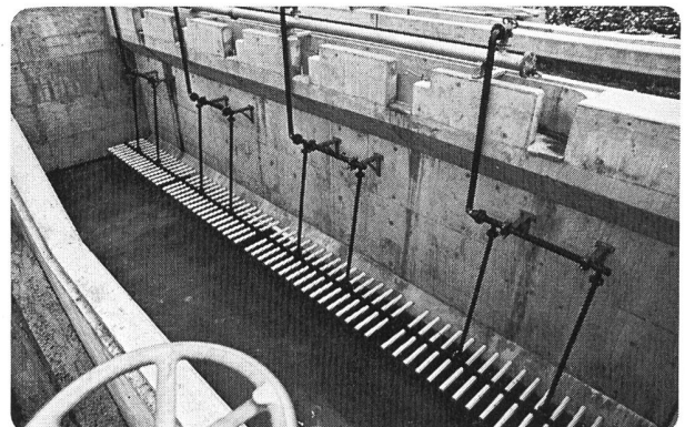
Ausschwenkbare Belüftungseinrichtung (ARA, Wartau/SG)
