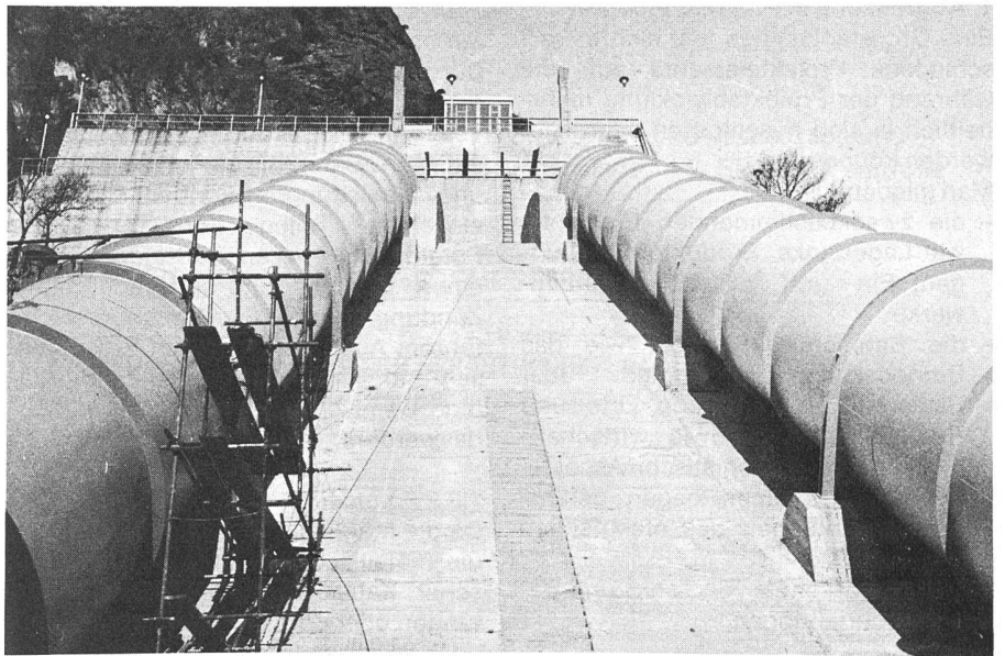
Abb. 3. Kraftwerk Säckingen, Anstrich der Wehranlagen. Vorbehandlung: Sa 3. Beschichtungsaufbau: Spritzverzinkung, 2× Vinoxink R, 2× Afratop A 70.
