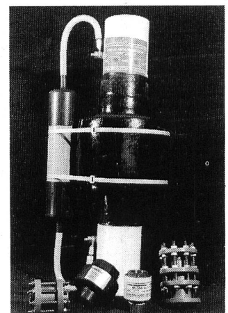
▼ Ziefle-Monobloc-Isolierstück mit aufmontiertem Überspannungsableiter. Auswahl von Ziefle-Rohrleitungsbauteilen.
