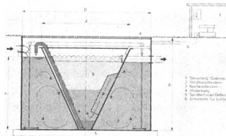
Abb. 2. Gruppenreinigungsanlage MWB: 1 Steuerung / Gebläse; 2 Belüftungsbecken; 3 Nachklärbecken; 4 Abdeckung; 5 Sandbett oder Ortbetonplatte; 6 Schutzrohr für Luftleitung.
