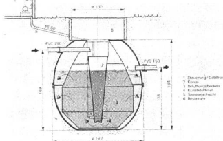
Abb. 3. Hauskläranlage MWB: 1 Steuerung / Gebläse; 2 Konus; 3 Belüftungsbecken; 4 Kunststoff-Filter; 5 Sammelschacht; 6 Betonrohr.
