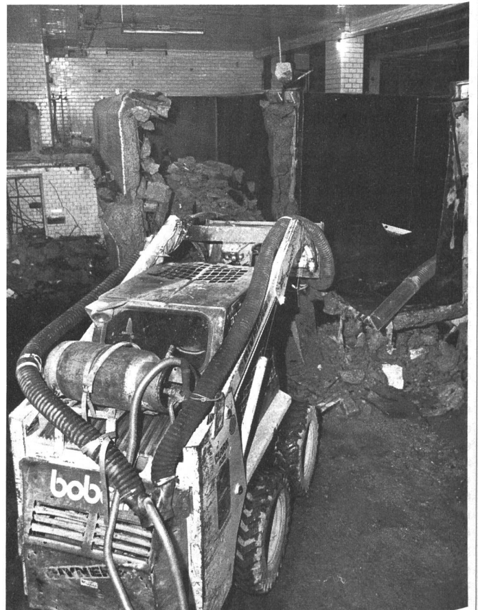
Zusätzlich zur Punktabmung am Abbruchhammer wird die Staubluft in der weiteren Umgebung über starke Saugrüssel zum Ventilationsaggregat abgeführt. Das Prinzip der gesteuerten Arbeitsplatzventilation bedingt, dass auch diese Absaugrohre immer möglichst nahe an die Staubquelle gebracht werden. Sie sind deshalb über flexible Schläuche an die feste Saugleitung angeschlossen.
