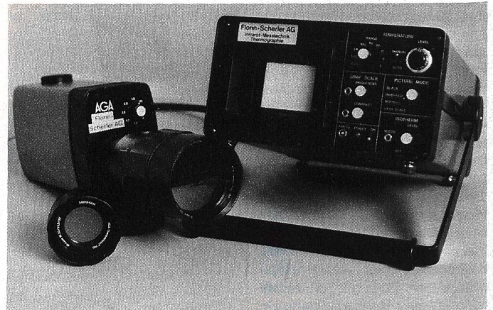
Abb. 5. Die Messausrüstung, bestehend aus Aufnahmeinheit und Monitor.
