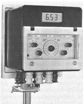
Vielfachmessgerät mit digitaler Anzeige Metravo 1D.
