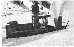
Einsatz der VF4 HM im Voralpengebiet. Arbeitsbreite wahlweise 2,3 oder 2,5 m.
