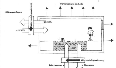
Wärmeverluste in Hallenbädern und Möglichkeiten zur Rückgewinnung.
