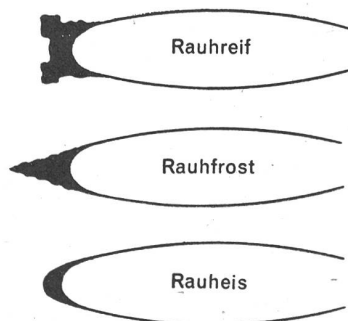
Bild 5: Grundformen der Vereisung: glasiger Überzug, große Haftfähigkeit, reißfährlicher weißer Ansatz mit großer Haftfähigkeit, weißer Ansatz, aber mit geringer Haftfähigkeit.
