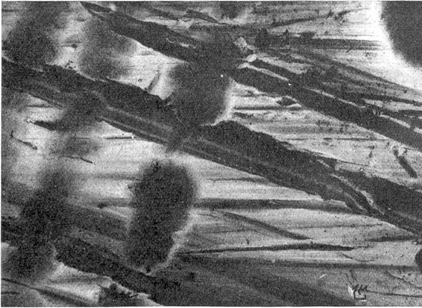
Bild 7: Oberfläche eines feingeschliffenen Stahls, aufgenommen mit einem Lack-Abdruck. Es ist eine Stelle wiedergegeben, die vorher mit einem mechanischen Rauigkeits-Prüfgerät abgetastet worden war. Die großen Abtastspuren, die als dunkle Flecken zu sehen sind, beweisen, daß die eigentliche Mikrostruktur der Oberfläche durch die Abtastung nicht erfaßt wird. (Vergrößerung 2500:1)
