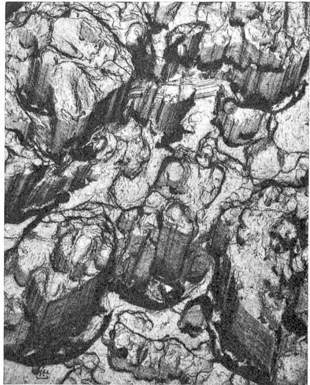
Bild 6: Präge-Abdruck von der Bruchfläche eines Stahlstiftes. Die Struktur der Bruchfläche gibt einen Einblick in die Gefügestruktur des Stahls, der in diesem Beispiel aus parallel gelagerten stäbchenförmigen Kristalliten besteht. (Vergrößerung 2500:1)
