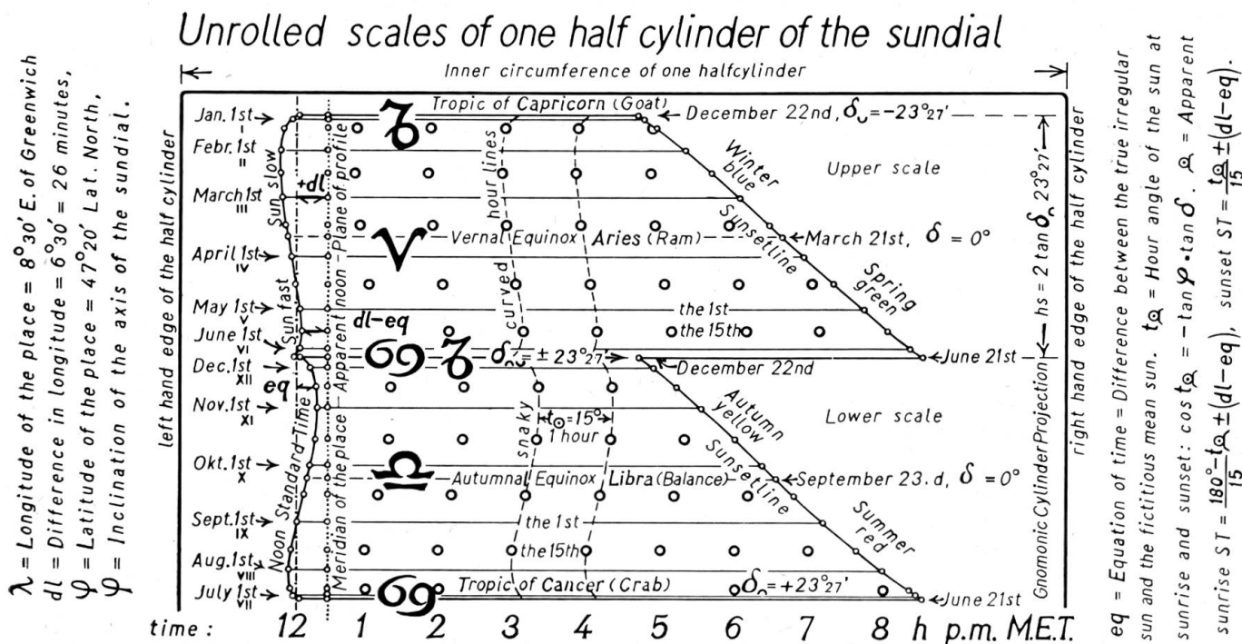
Abb. 7. Zifferblatt der Gnomonischen Sonnenuhr. (Westliche Zylinderhälfte)
